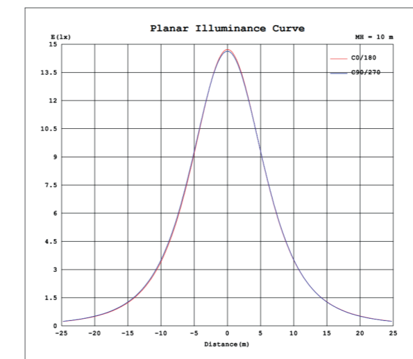
LVK Kegel
