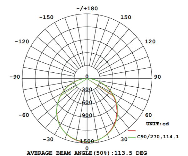
LVK Polar
